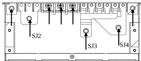
Okablowanie wejściowe 3:1 z podwójnym źródłem zasilania
