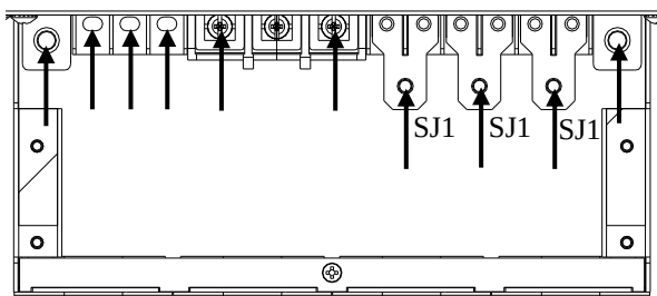
Okablowanie wejściowe 3:3 z jednym źródłem zasilania
