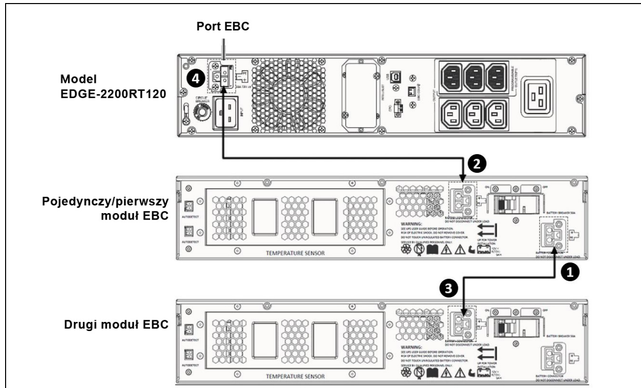
Rysunek 3.4 Podłączanie akumulatorów zewnętrznych
